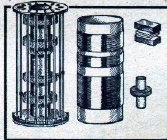
Ganz links eine moderne Industrie-Luftspule: Die Spule des deutlichen Volksempfängers. Daneben eine typische Zylinder-Spule. Rechts oben die bekannteste Eifenkernspule für Baßler zum Selbstwickeln. Darunter die Form der Eifenkernspulen, die man in den neuesten Geräten des Konzerns Telefunken-Siemens-AEG finden wird.
