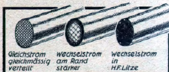
Zum Verständnis der „Hautwirkung“ (Skinneffekt).
