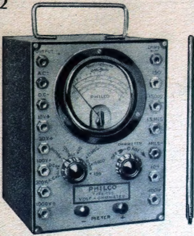
Rechts: Ein scharfkantiger Schraubenzieher aus Isoliermaterial mit Stahleinsatz, mit dem man auch im eingefalteten Gerät arbeiten kann.
