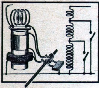
Eine vollständige Empfängerspule besteht aus drei Teilen, die durch einen „Wellenschalter“ (in moderner Ausführung als sog. Nockenhalter) kurzgeschlossen werden, soweit sie zum Empfang des gerade eingestellten Wellenbereichs nicht nötig sind.
