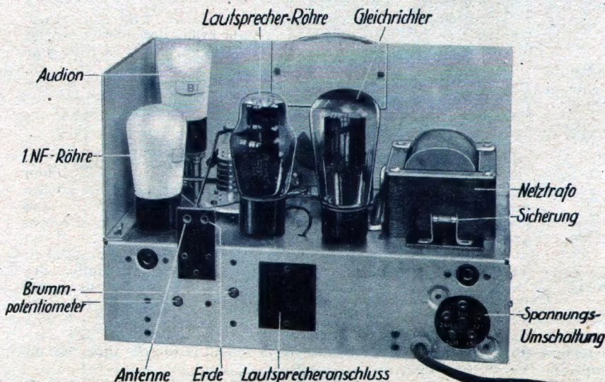
So sieht der UKW-Spezialempfänger aus, wenn man die Rückwand abnimmt.
